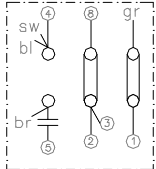
Anschlußbild im Motor
